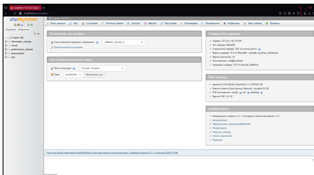
Рисунок 5. Страница phpMyAdmin
